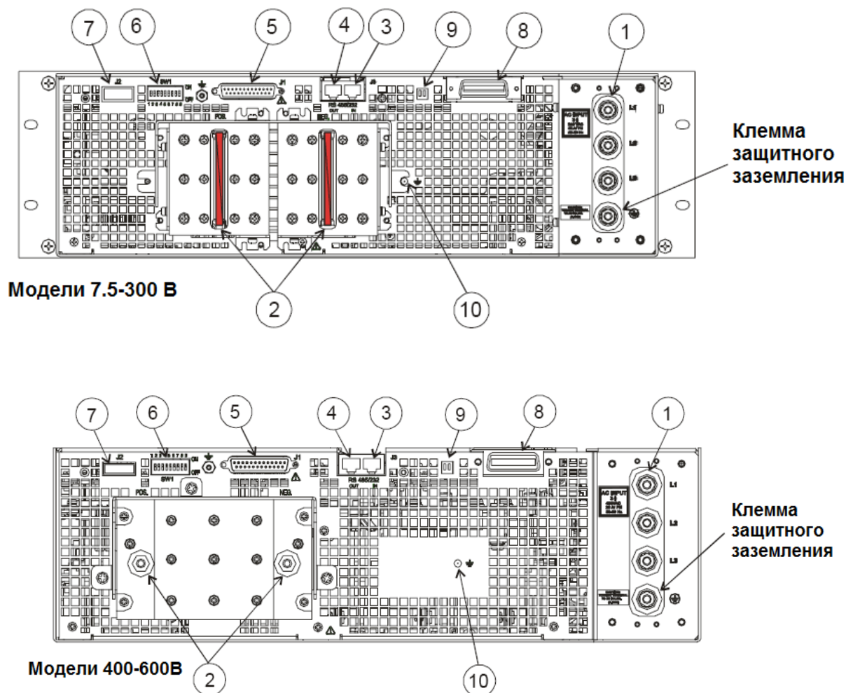
Рис.4-2: Соединительные разъемы и органы управления задней панели
