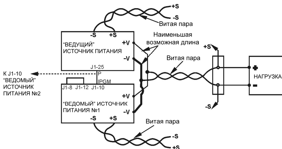
Рис.5-5: Параллельное соединение в режиме внешнего контроля
