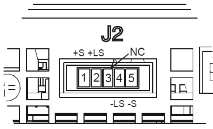
Рис.3-9: Расположение сенсорного разъема
