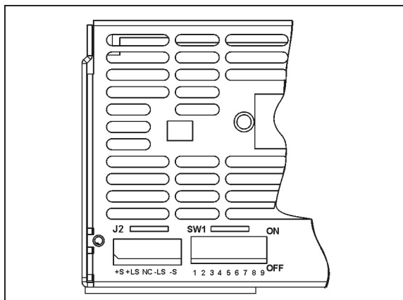
Рис.3-14: Расположение сенсорного разъема
