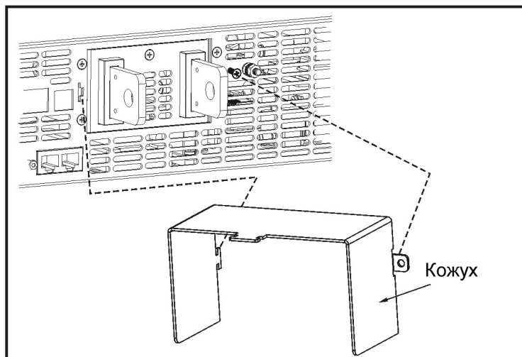
Рис. 3-7: Монтаж кожуха
