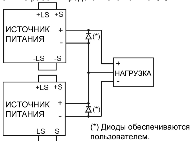
Рис.5-3: Последовательное соединение для получения положительного/отрицательного выходного напряжения
