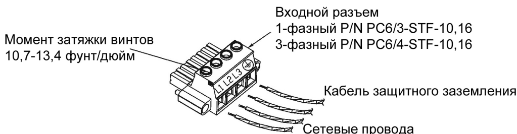
Рис.3-3: Входной разъем (на рисунке трехфазный)
