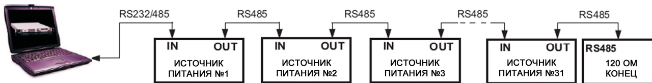
Рис. 7-5: Подсоединение нескольких источников питания через RS232/485
