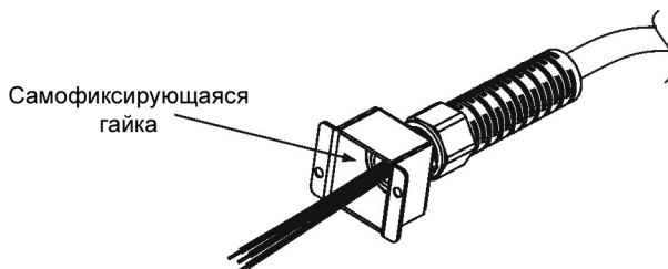
Рис.3-2: Зачищенные провода, установленные в разгрузочной муфте
